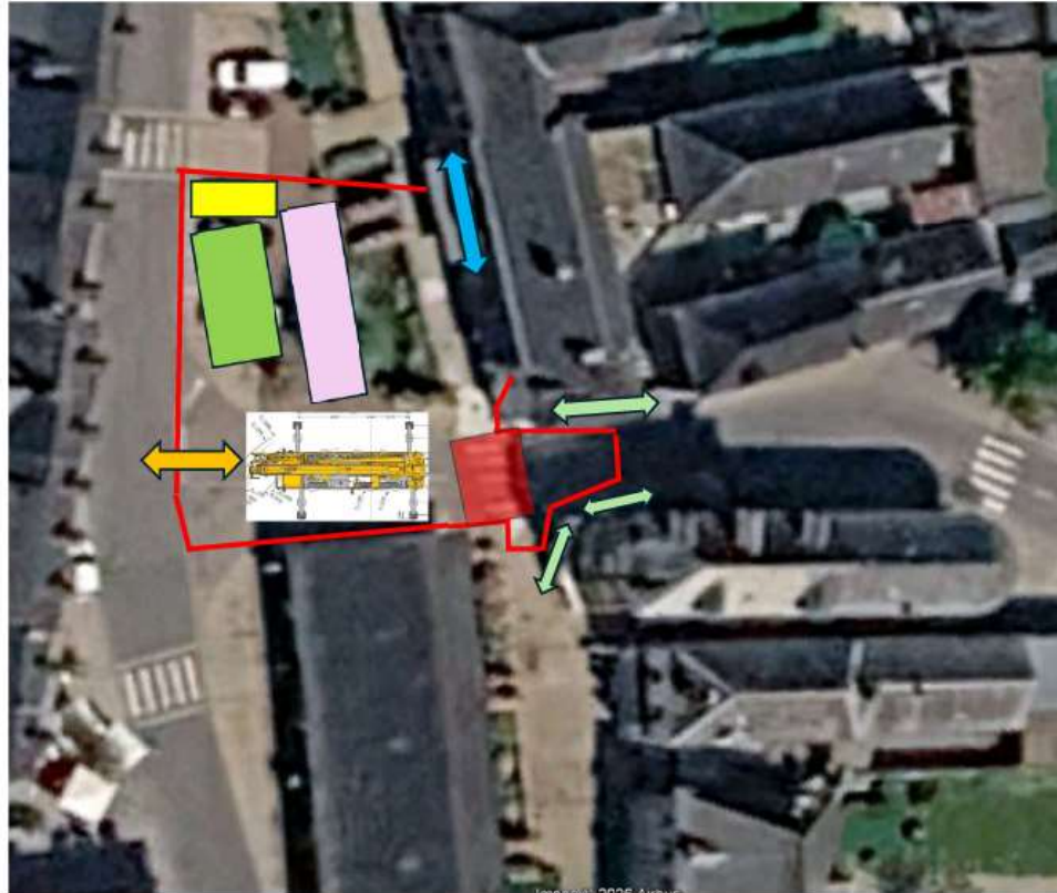
Plan d'installation de chantier – OA Clères
